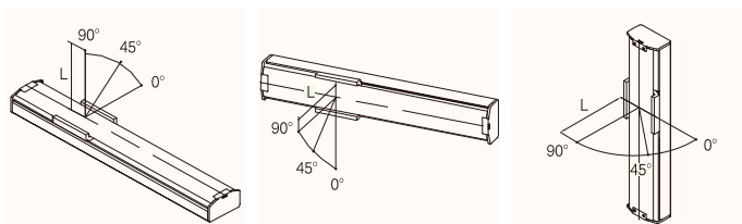
水平安裝應用(單位:mm) Horizontal use
