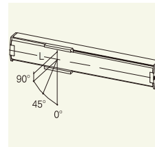
牆面安裝應用 (單位:mm) Wall installation use
